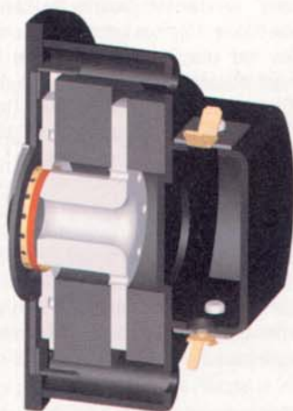
Wunderwerk der Technik: Die extrem verzerrungsarme Keramikkalotte KE25SC von Visaton beinhaltet sogar ein RC-Glied
