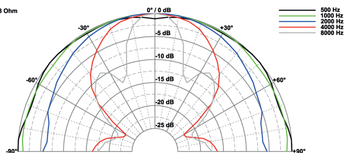
DK 121 - 8 Ohm
